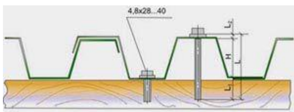
Рис.5. Крепление кровли из профнастила: L = H + L1 + L2 , (мм) Где Н - высота профиля профнастила, мм L1 = 25...30 мм - длина резбовой части, которая входит в деревянную обрешетку L2 = 4 мм - толщина уплотнительной прокладки и шайбы
