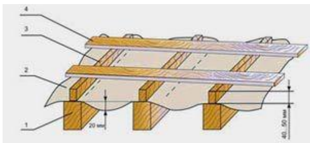
Рис.3. Укладка гидроизоляционной плёнки и обрешётки: 1 - стропильная нога; 2 - гидроизоляция; 3 - стропильная планка (брус конобрешетки); 4 - обрешётка
