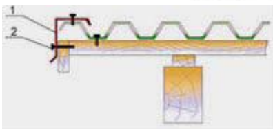
Рис.7. Крепление ветровой планки: 1 - «ветровая» планка; 2 - саморез
