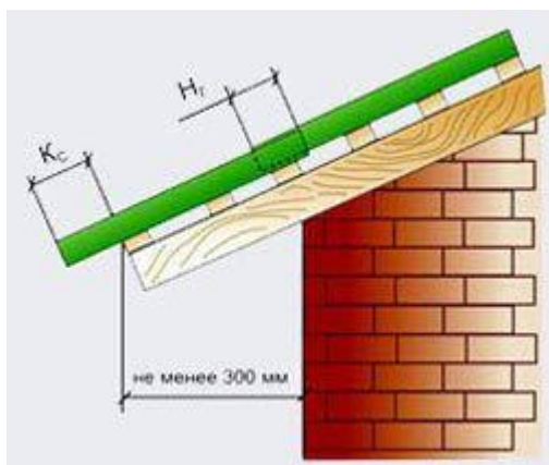
Рис.4. Карниз кровли из профнастила: Нг - нахлест горизонтальный; Кс - карнизный свес. Для НС-8, НС-10, НС-20, С-21 - карнизный свес - не менее 50-100 мм. Для НС-35, С-44, Н-60, Н-75 - карнизный свес - не менее 200-300 мм..
