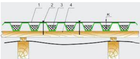
Рис.10. Крепление конька: 1 - конёк; 2 - саморез; 3 - уплотнитель коньковый; 4 - обрешётка; К - вентиляционный зазор
